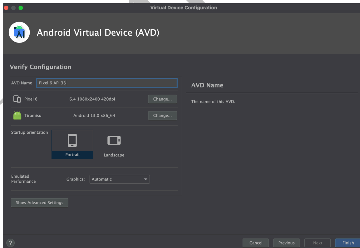
Рисунок 2.14 – Экран конфигурирования эмулятора
