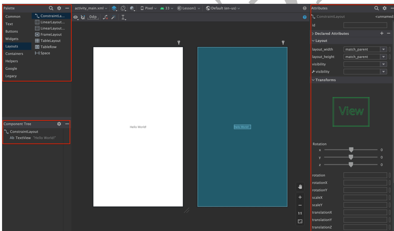
Рисунок 3.4 – Экран редактирования « layout » файла.
