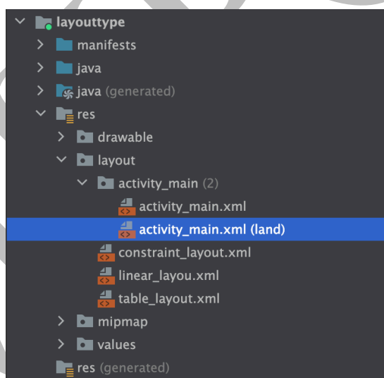
Рисунок 5.3 – Каталог файлов разметки
